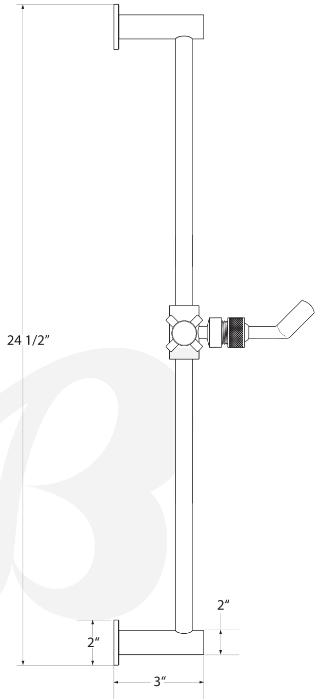
Slide Bar - P11301xx
