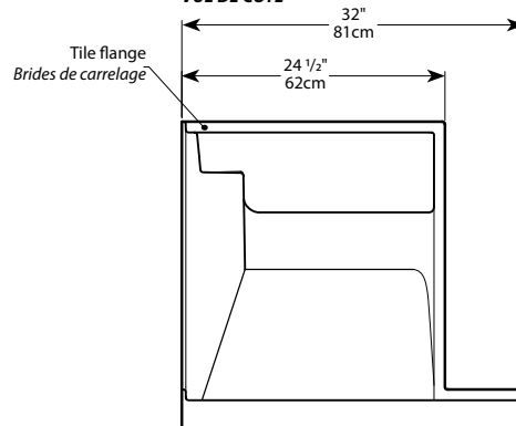
TOP VIEW VUE DE CÔTÉ
