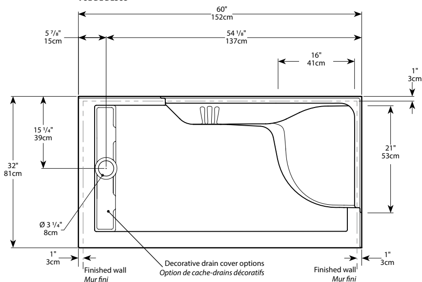
TOP VIEW VUE DE DESUS
