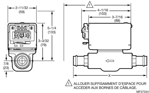
Fig. 2. Dimensions (V8043F). Mesures en po (mm). Voir le Tableau 1.
