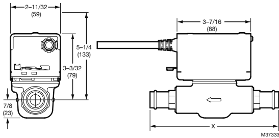
Fig. 1. Dimensions (V8043A, V8043E). Mesures en po (mm). Voir le Tableau 1.
