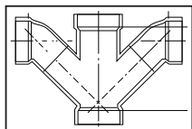
Doble Combinación WYE / 1/8 Curva
